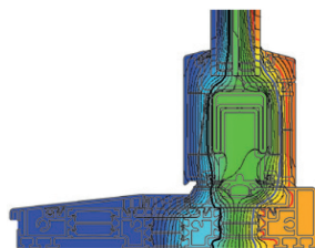
Isotermenvverloop CT70 HS
