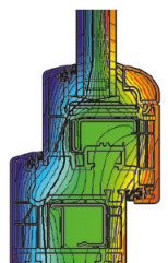
Isotermenverloop CT70 Accent
